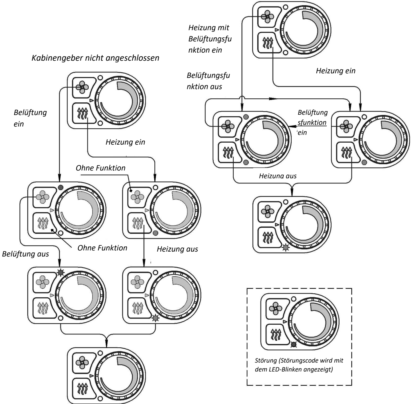
Funktionsschema der Bedienungskonsole
