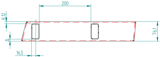
SEZIONE A-A
