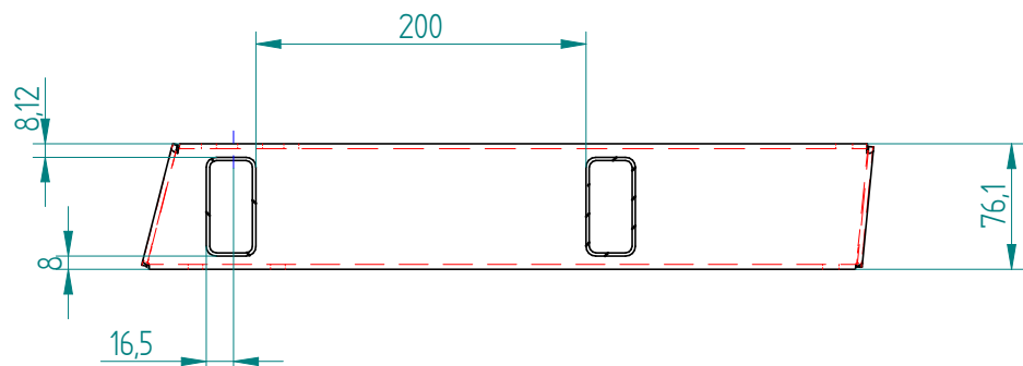
SEZIONE A-A
