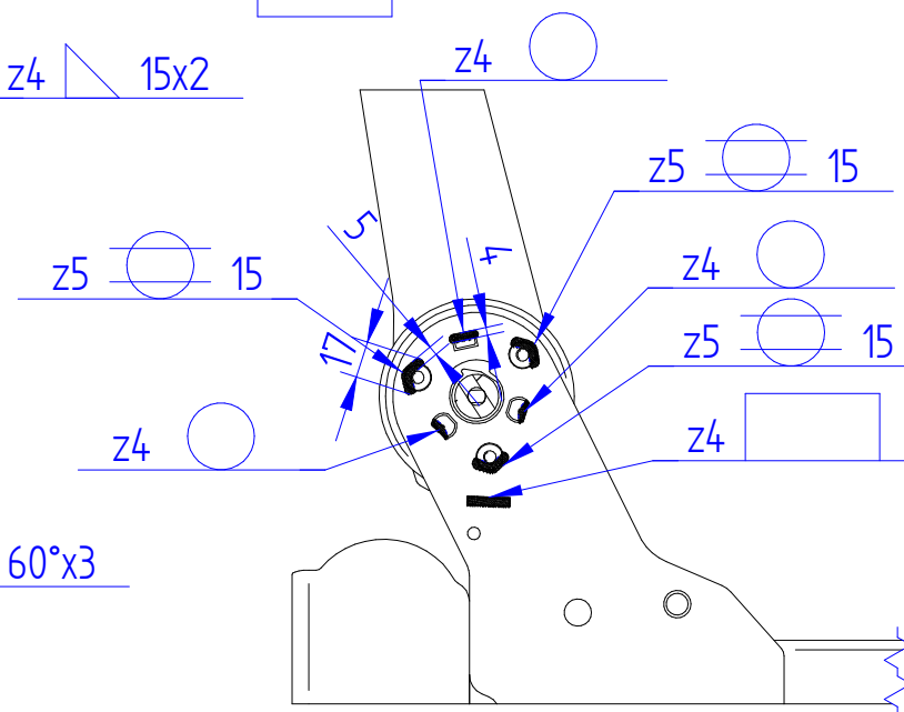
SEZIONE E-E
