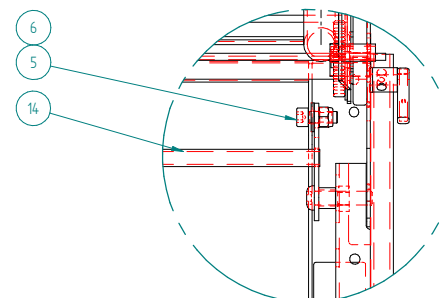
DETTAGLIO C
