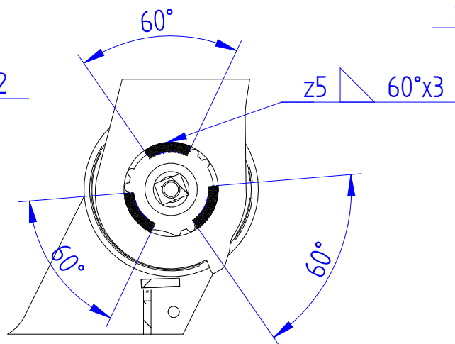
SEZIONE G-G
