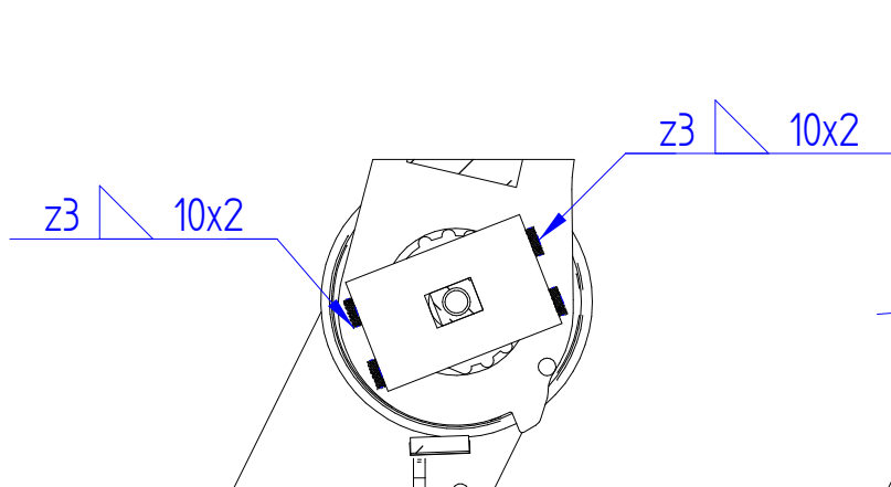
SEZIONE F-F
