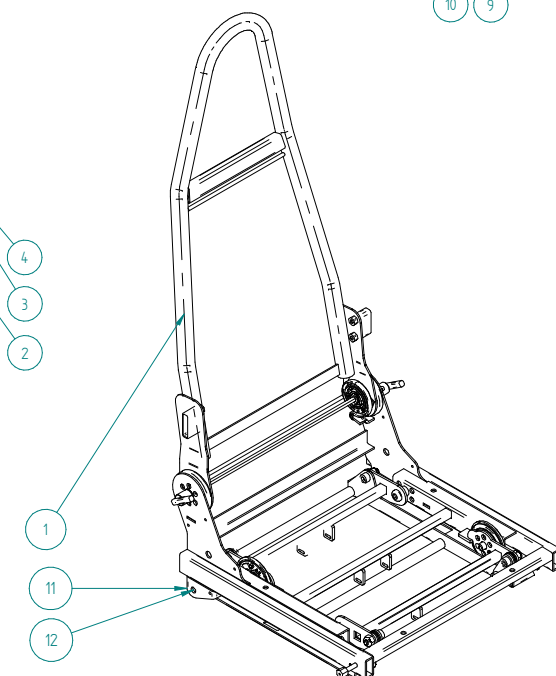
DETTAGLIO C
